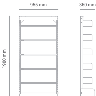
Estante ESBS
