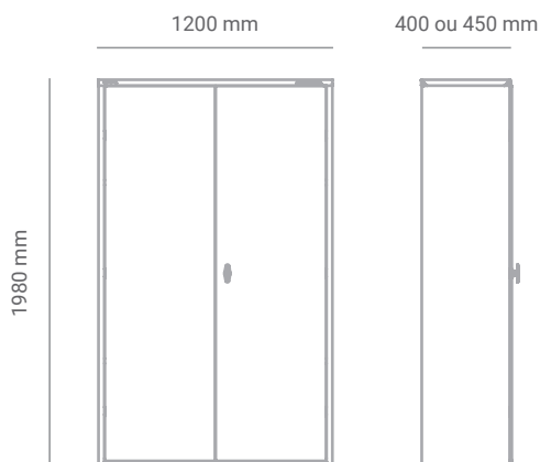
Armário Aço Duas Portas PA120
