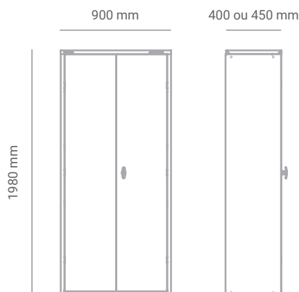
Armário Aço Duas Portas PA90
